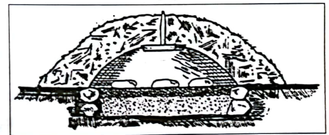
Abb. 6 Hebräischer Backglockenherd
