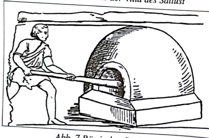
Abb. 7 Römischer Backofen
