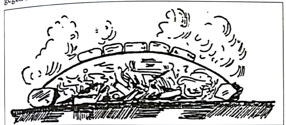
Abb. 5 Hebräischer Fladenofen
