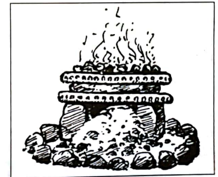
Abb. 1 Tonteller-Fladen-Backgeschirr
